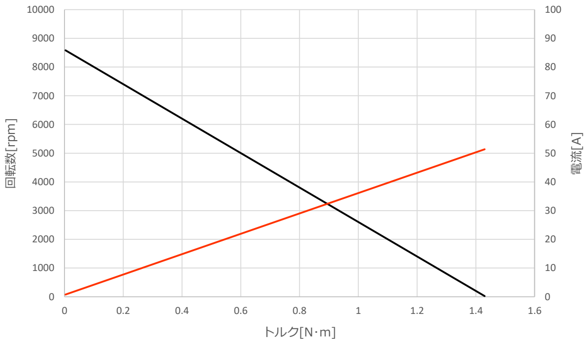
■特性図 Characteristics
